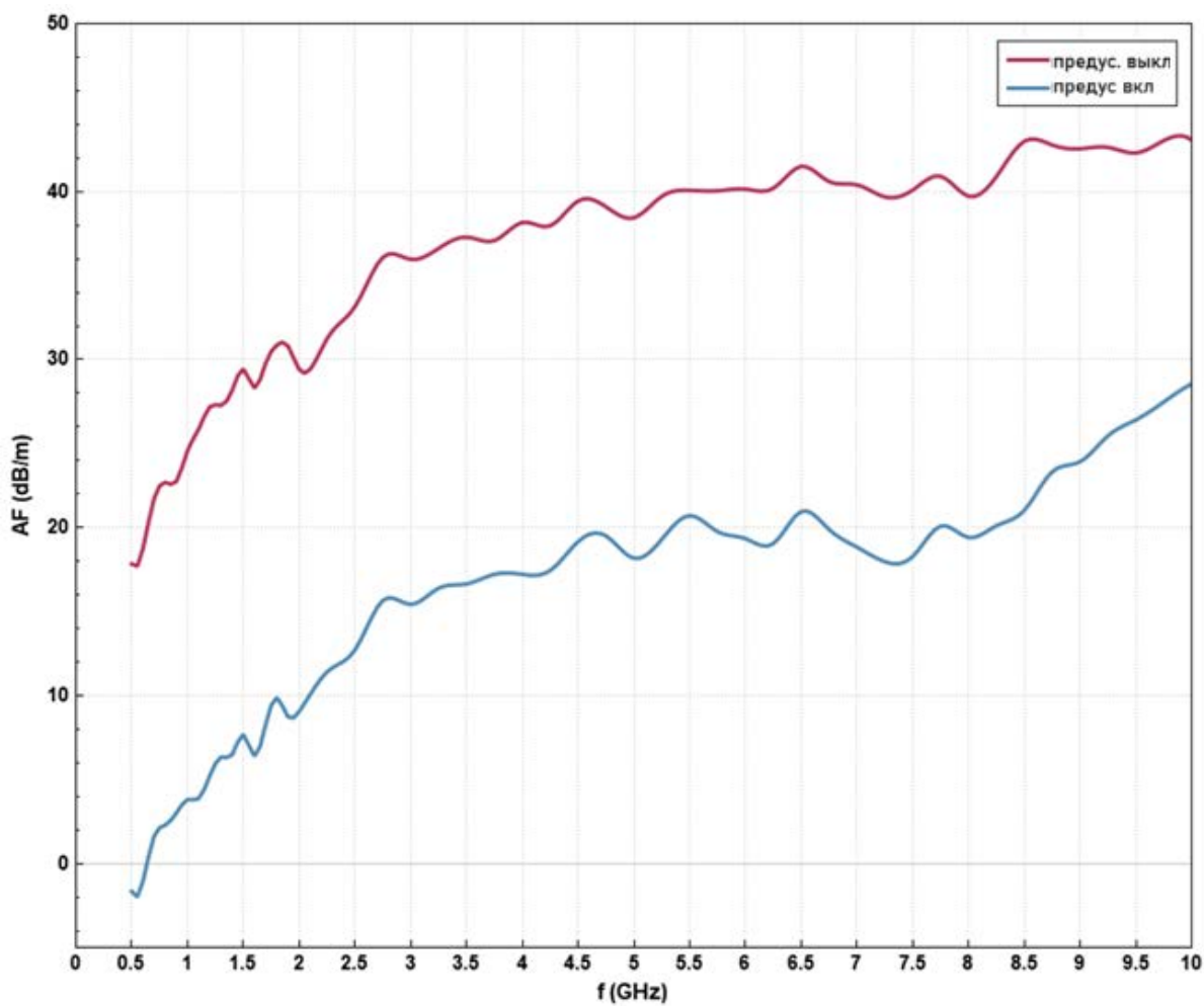
АНТЕННЫЙ ФАКТОР
